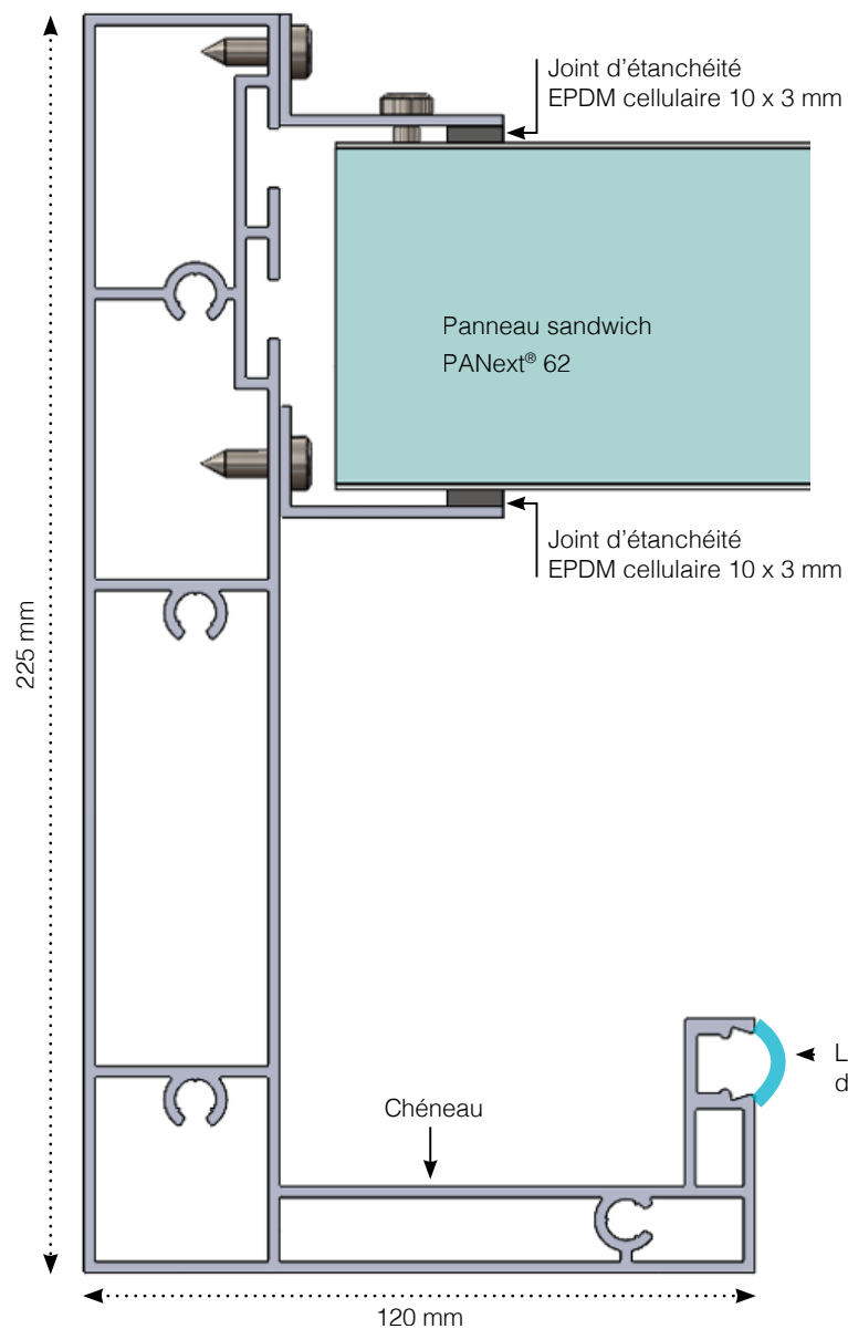
COUPE VERTICALE CÔTÉ DU PANNEAU EN POSITION HAUTE
