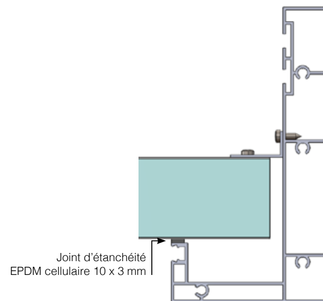
COUPE VERTICALE CÔTÉ ÉVACUATION EAU
