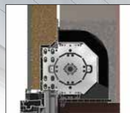
Pose en demi linteau
