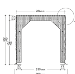
Parement extérieur ciment (std.)
