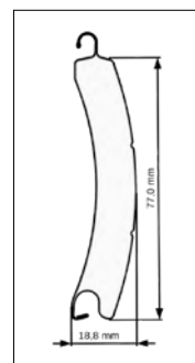
Lame 77 jusqu'à larg. 6000 mm
