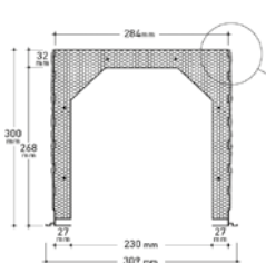
Parement extérieur ciment (std.)
