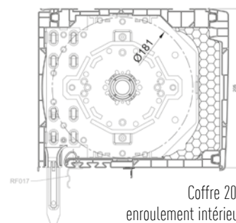
Coffre 168 enroulement intérieur
